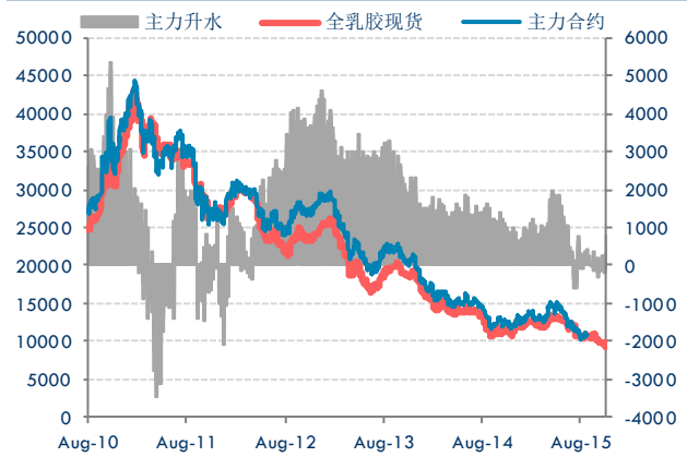
期现价差
