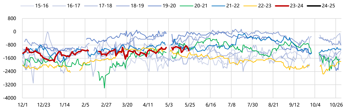
图表 124: 价差: 国产标二-全乳老胶 11合约周期 (元/吨)
