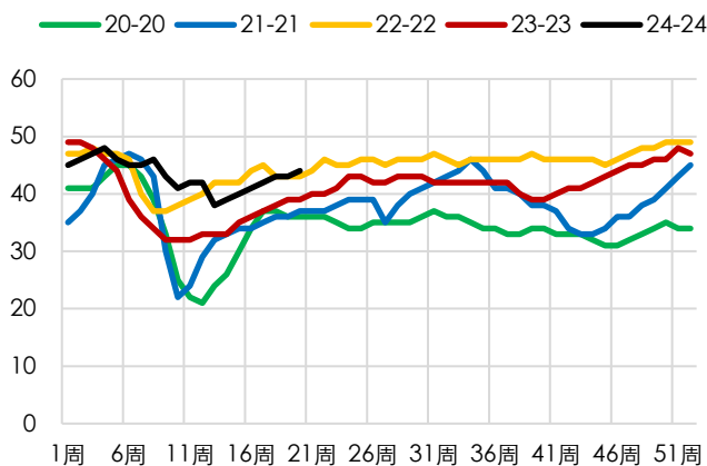
图表 218: 国内全钢轮胎产线成品库存 (天)
