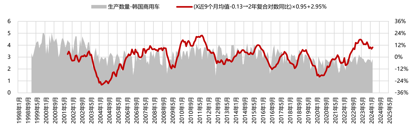
图表 204：生产数量-韩国商用车（万辆）
