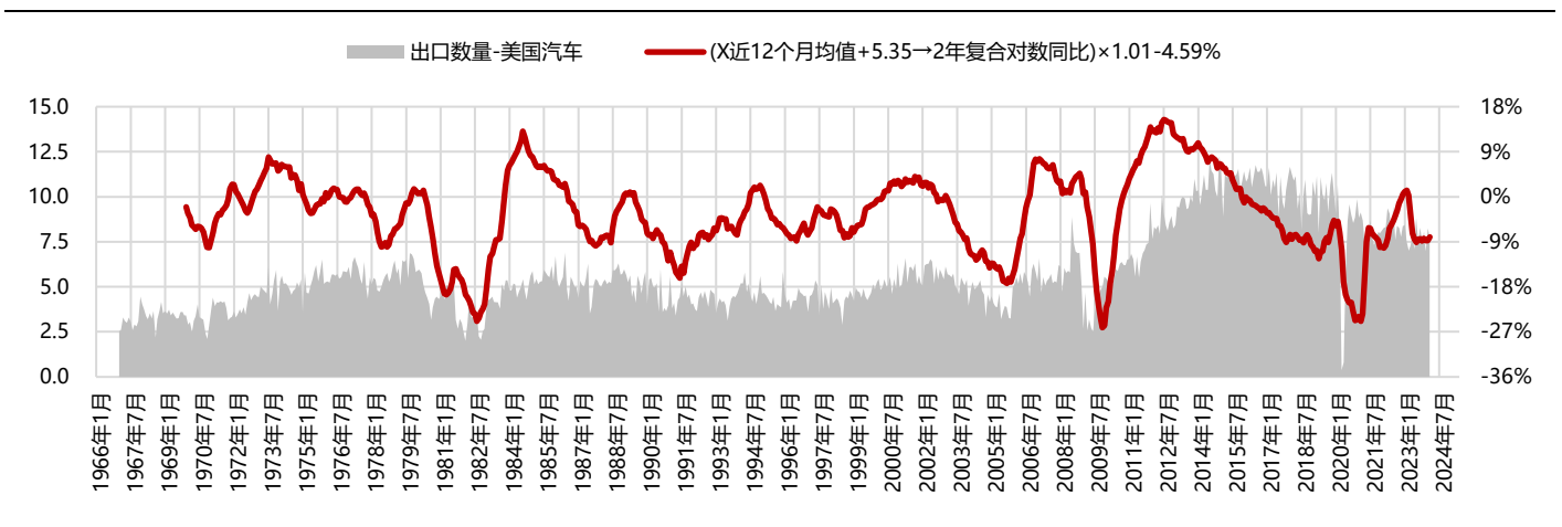
图表 196：出口数量-美国汽车 (万辆)
