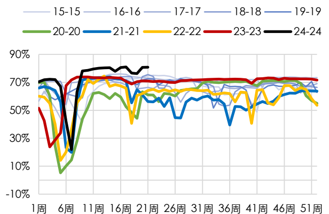
图表 213：国内半钢轮胎开工率
