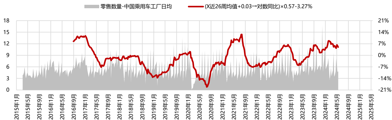
图表 236: 乘用车厂家当周日均零售量 (万辆)
